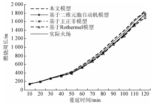
图5 火场周长对比
