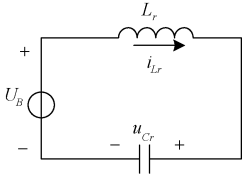
图 4 模式 5 的谐振腔等效电路
